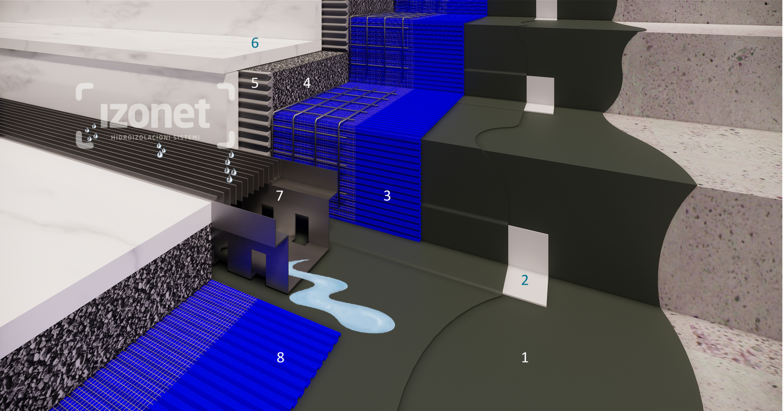
1. ARDEX 8+9 hidroizolacija 2. ARDEX SK 12 traka 3. AQUADRAIN® SD drenažni sloj 4. ARDEX A10 + kvarcni pijesak granulacije 3.0 - 5.6 mm 5. ARDEX FB9L ljepljivo za kamen/keramiku 6. keramičko/kameno završno popločanje 7. AQUADRAIN FLEX linijski slivnik 8. AQUADRAIN® EK drenažni sloj
